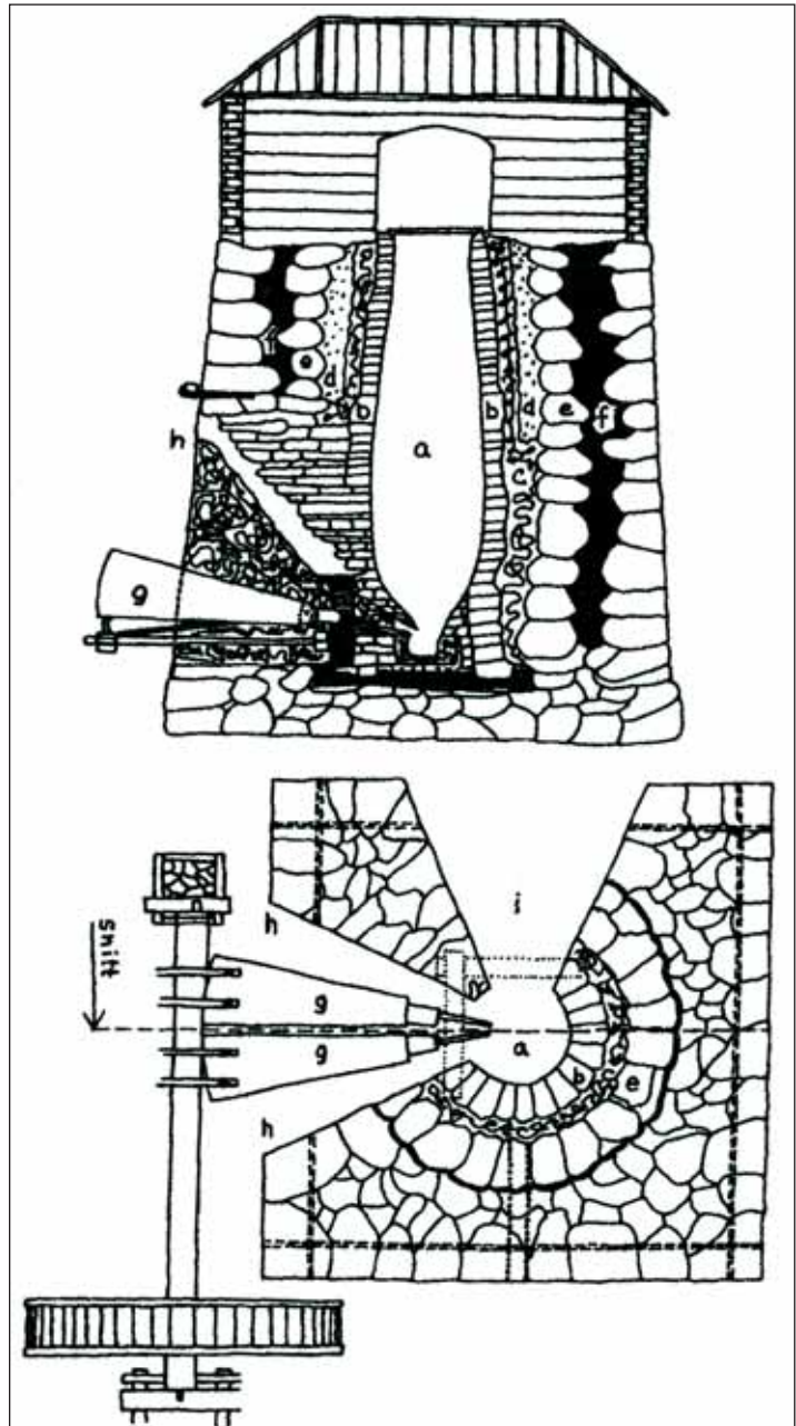
Masovn av vallonsk type (etter Rinman: Bergverks-Lexicon) a: pipe, b: ildfast sandstein, c: bakmur, d: sandfylling, e: ringmur, f: fylling av gråstein og leire, g: to store belger (for å oppnå høy temperatur), h: belgbryst.
