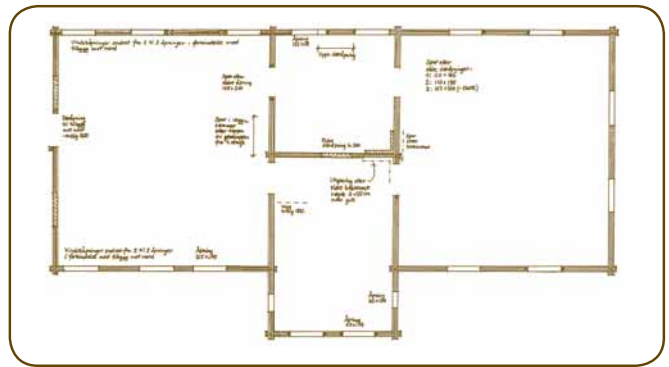
Plan over annen etg.
