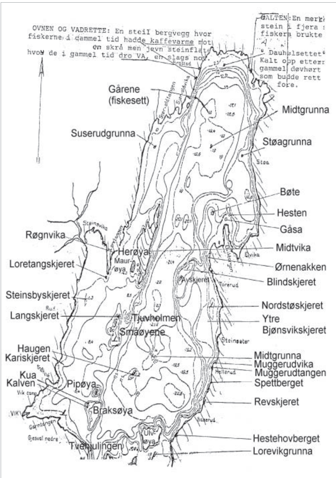
Dybdekart for Steinsfjorden med navn på fiskeplasser, grunner og øyer.
