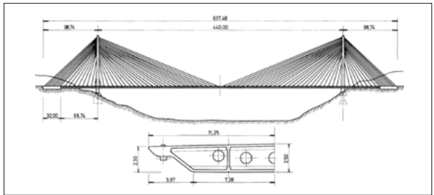
Barrios de Luna, Spania, skråstagbro, bygget av Brobyggeren.
