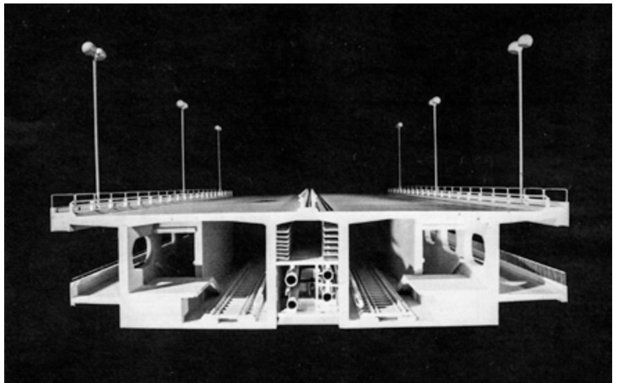
Tverrsnitt av Neue Reichsbrücke.
