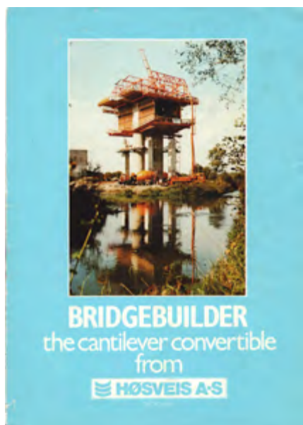
Forsiden av brosjyren til Høsveis viser bygging av Orwell Bridge, England. Cantilever = frittframbyggbro.
