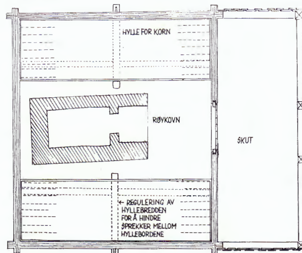
Tegninger: Plan og snitt.
